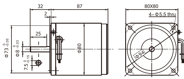
图9 80YS25 (25W) 交流三相电动机 Three-phase AC Motor
