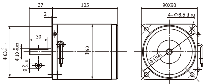
图10 90YS40 (40W) 交流三相电动机 Three-phase AC Motor
