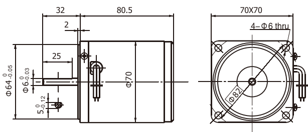
图8 70YS15 (15W) 交流三相电动机 Three-phase AC Motor
